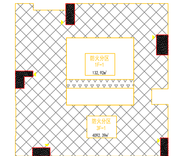
防火分区示意图
