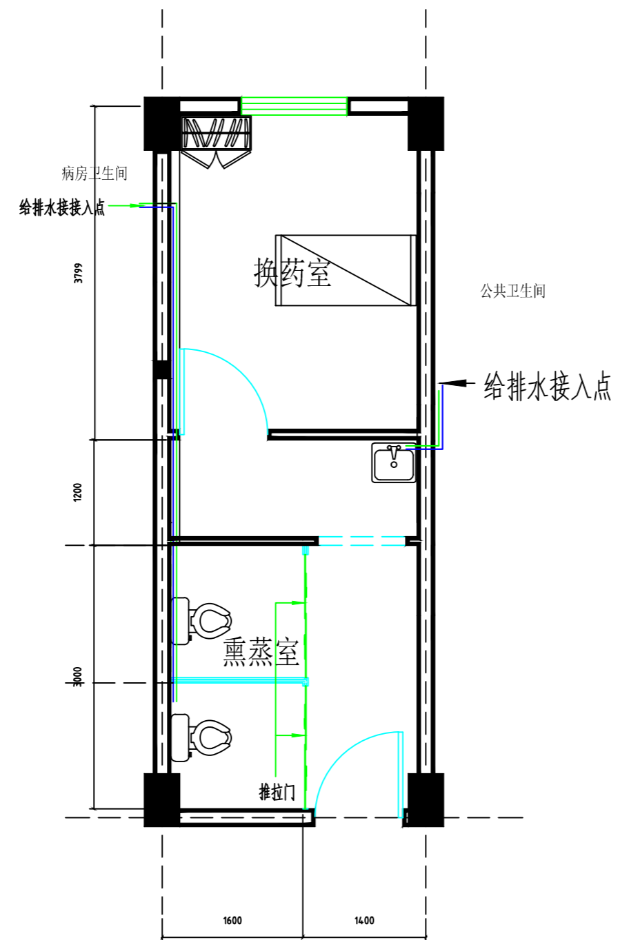
水施图
