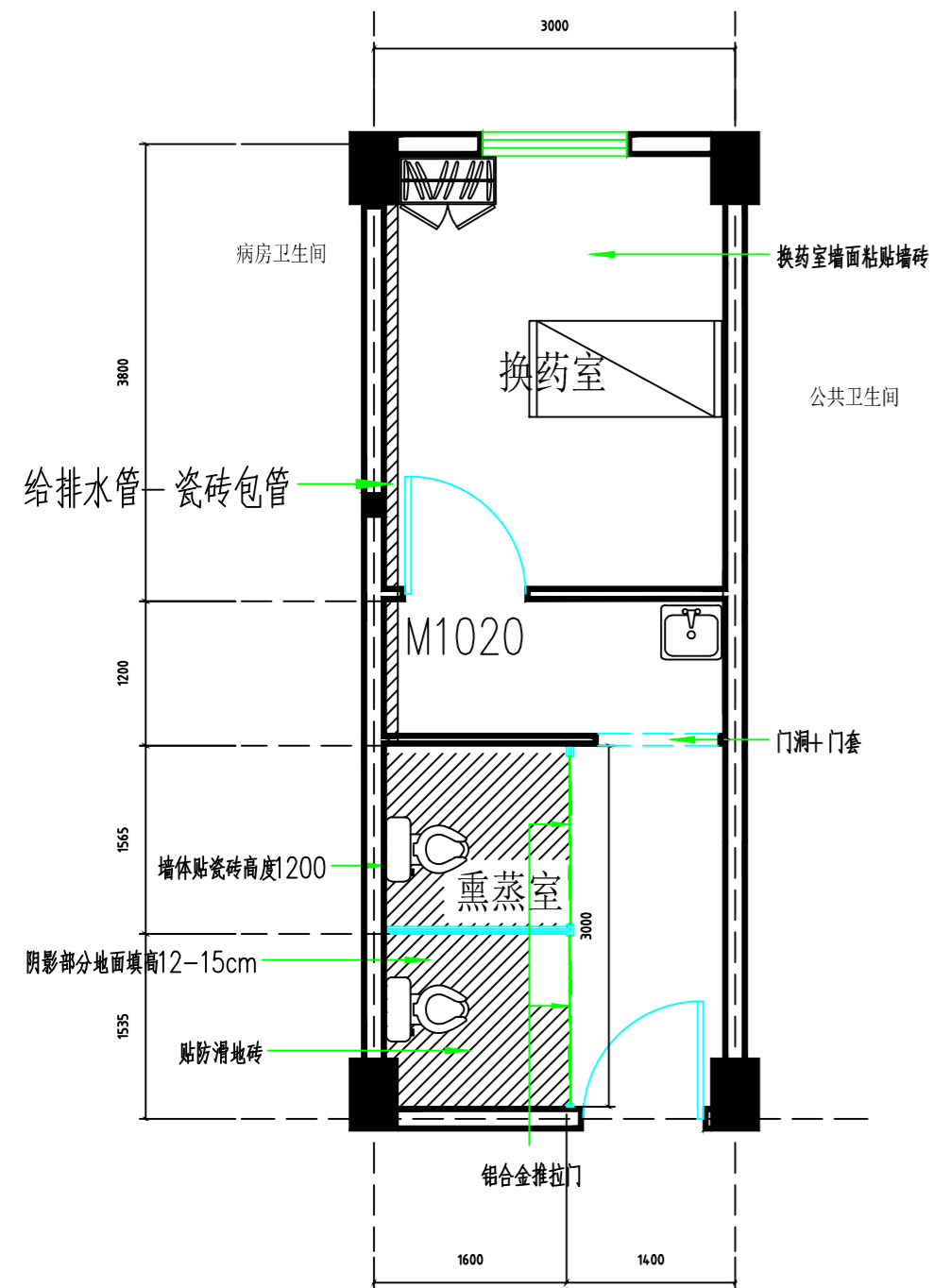
建施图
